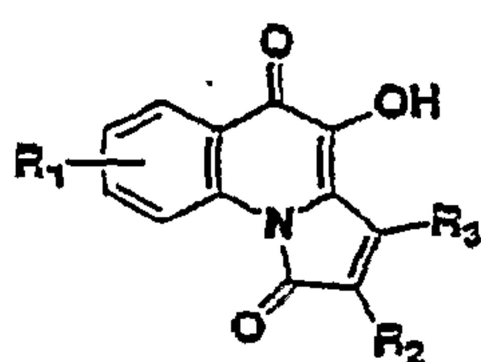
Pyrrolo[1,2-a]quinolines and Isoindolo[2,1-a]quinolines
