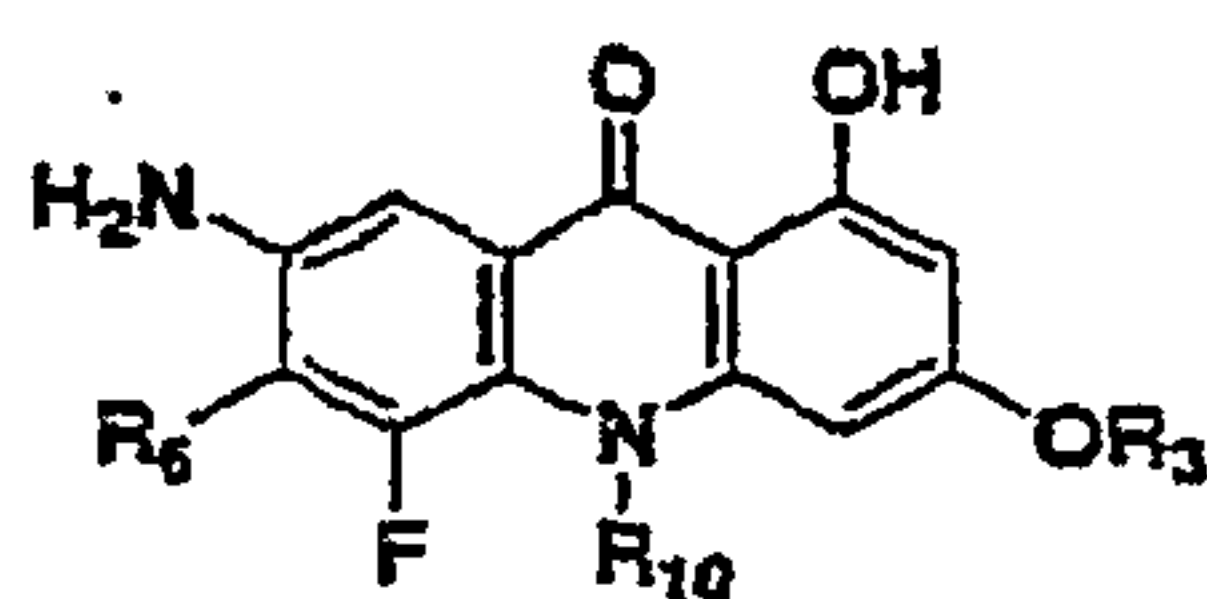
1-Hydroxy-7-amino-9-acridones
