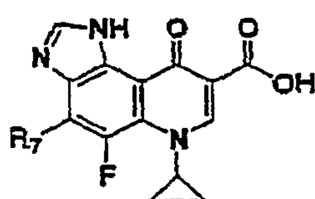
Pyrroloquinolones and Pyrazoloquinolones
