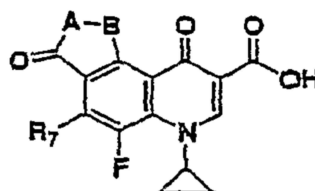
Pyrroloquinolones and Pyrazoloquinolones
