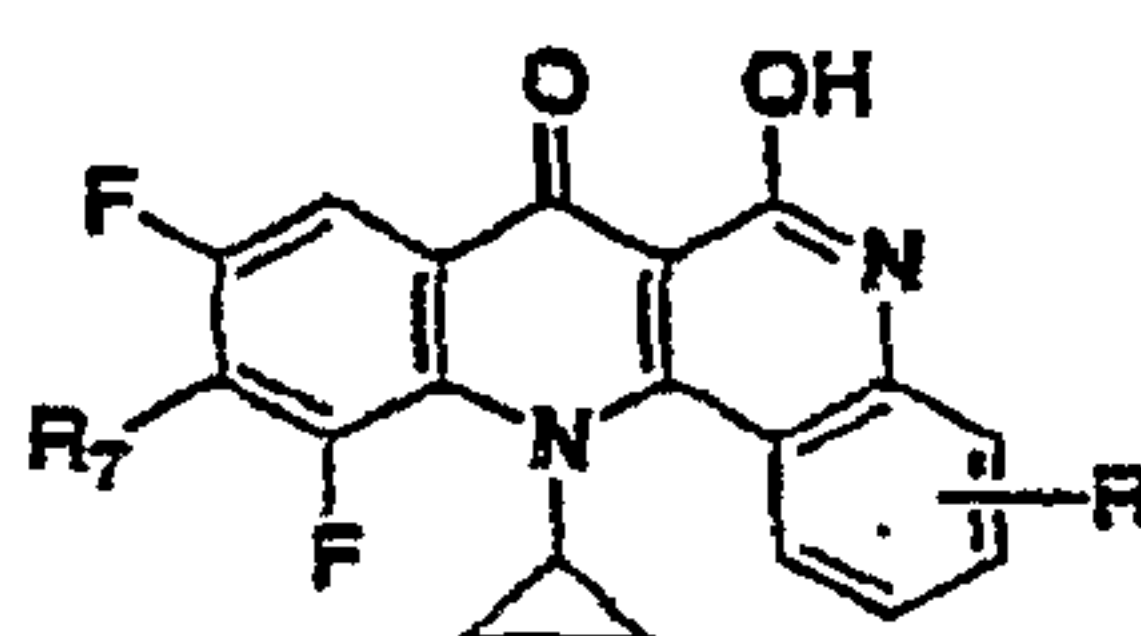
Dibenzo[1,5]naphthyridiones
