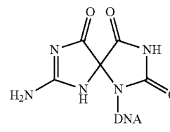
spiroiminodihydantoin Sp
