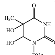
thymine glycol (cis & trans)
