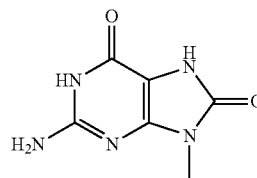
8-oxoguanine
