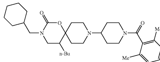
CF_3CO_2H
