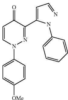
1-(4-Methoxyphenyl)-3-(1-phenyl-1H-pyrazol-5-yl) pyridazin-4(1H)-one
