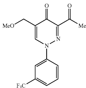
3-Acetyl-5-(methoxymethyl)-1-[3-(trifluoromethyl)phenyl]pyridazin-4(1H)-one
