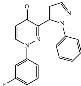
1-(3-Fluorophenyl)-3-(1-phenyl-1H-pyrazol-5-yl) pyridazin-4(1H)-one
