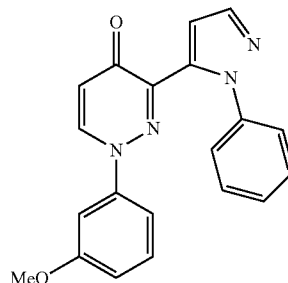
1-(3-Methoxyphenyl)-3-(1-phenyl-1H-pyrazol-5-yl)pyridazin-4(1H)-one
