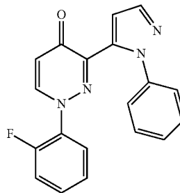
1-(2-Fluorophenyl)-3-(1-phenyl-1H-pyrazol-5-yl) pyridazin-4(1H)-one
