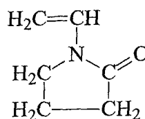
2-vinylpyrrolidone
