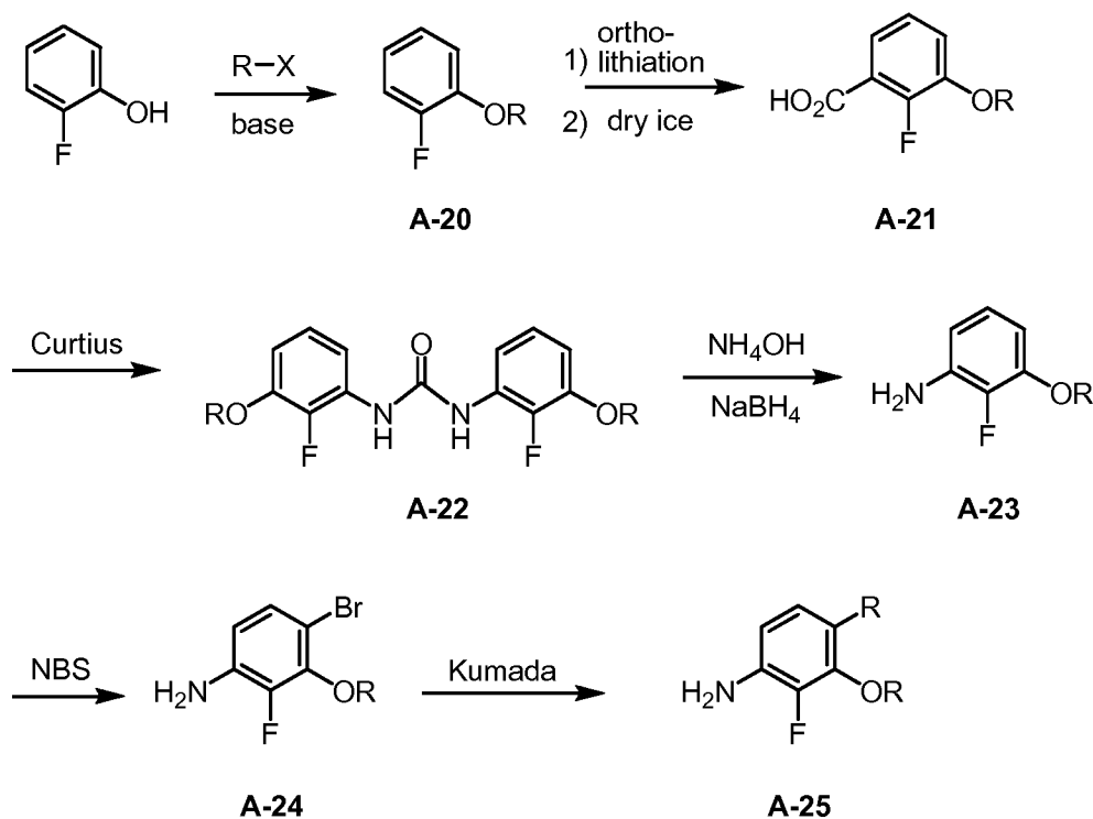
Scheme (IV)
