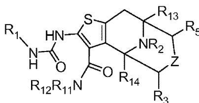
Formel (I) ;
