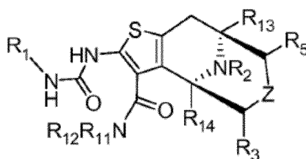
Formule (Ib).
