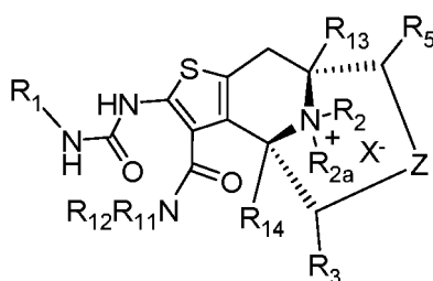
Formula (IIa);
