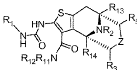
Formule (Ia) ;
