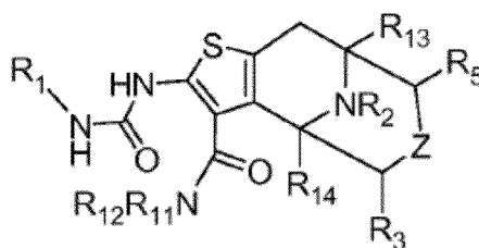
Formule (I) ;
