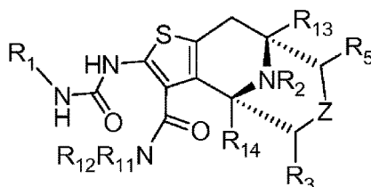
Formel (Ia);
