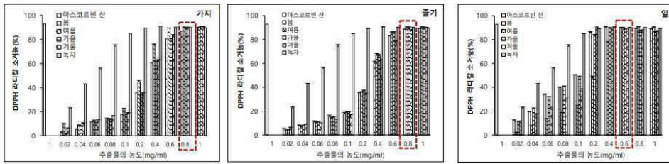
DPPH
