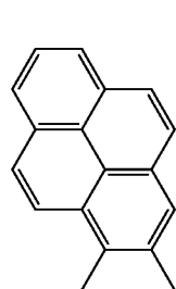
1,2-Pyr
