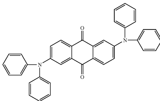
Int-3
