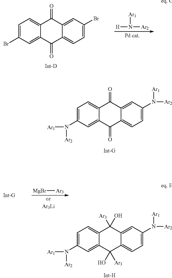
Scheme III:
