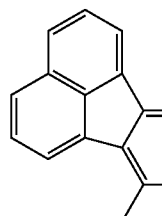
7,8-FlAn
