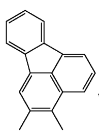
2,3-FlAn
