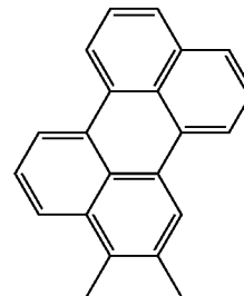
2,3-Per
