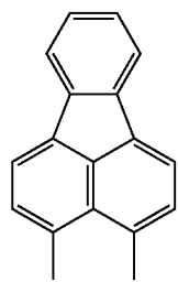
3,4-FlAn
