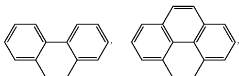
2,2'-BP
