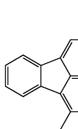
1,2-FlAn
