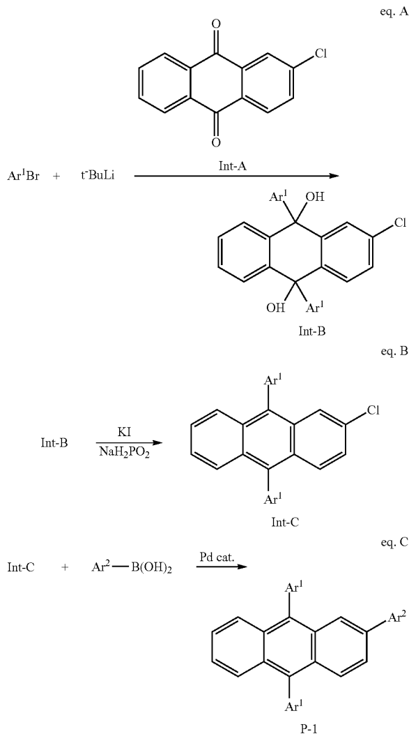
Scheme I:
