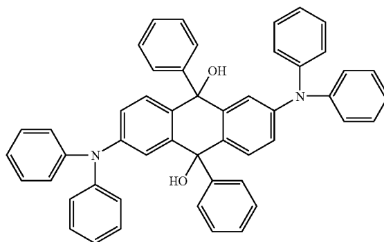
Int-4
