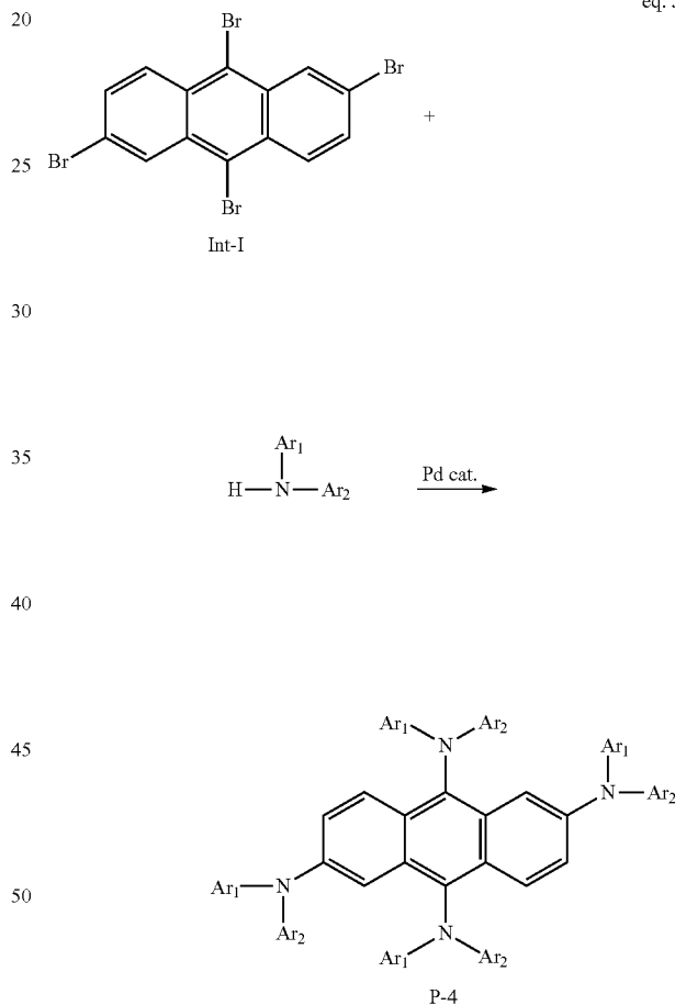
Scheme IV:
