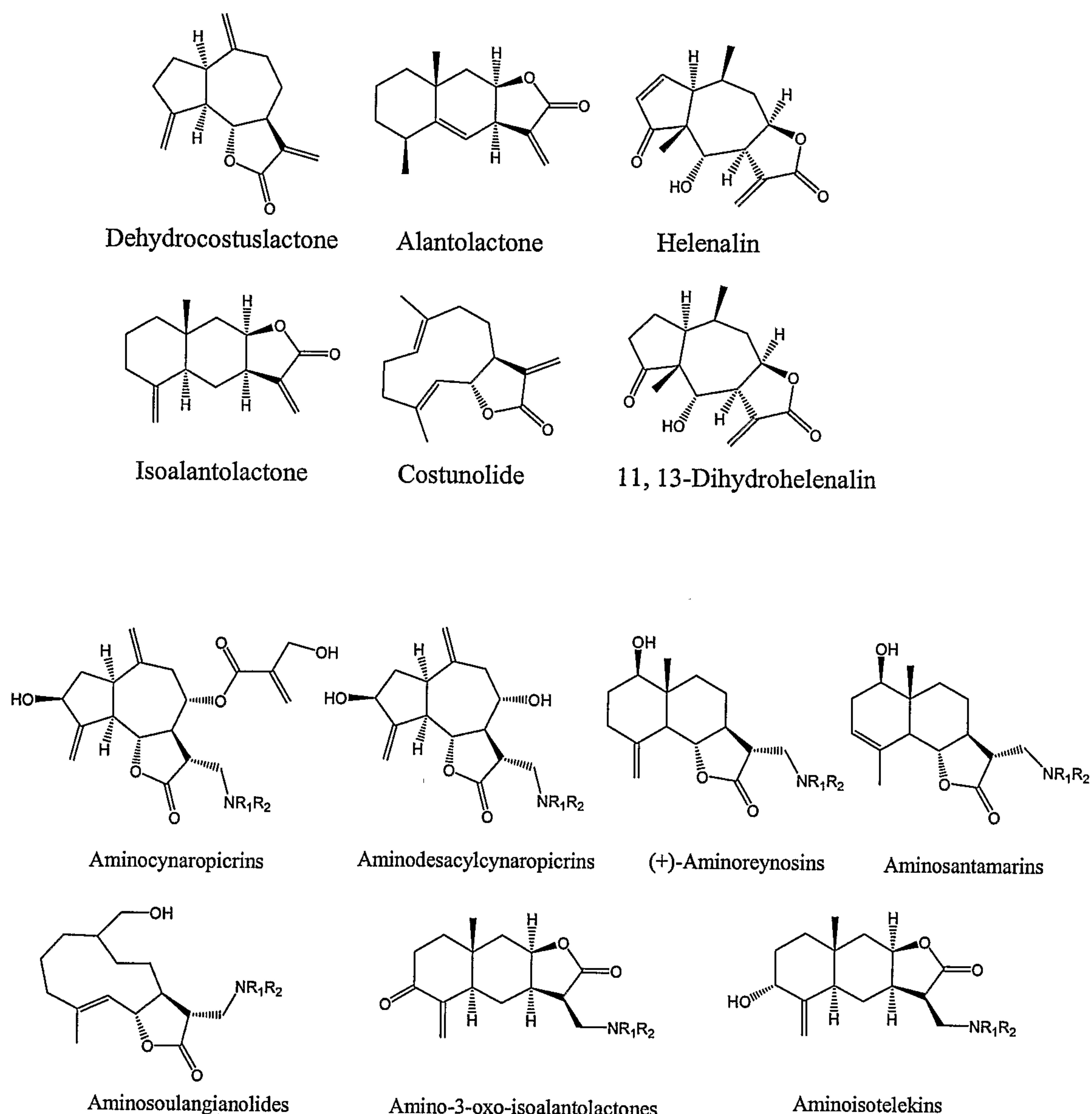
Scheme VI
