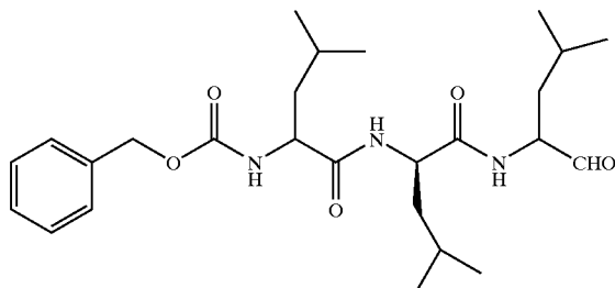
Z-Leu-Leu-Leu-CHO
