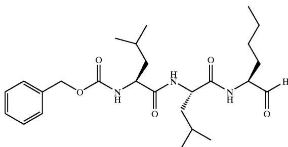
Z-Leu-Leu-Nva-CHO
