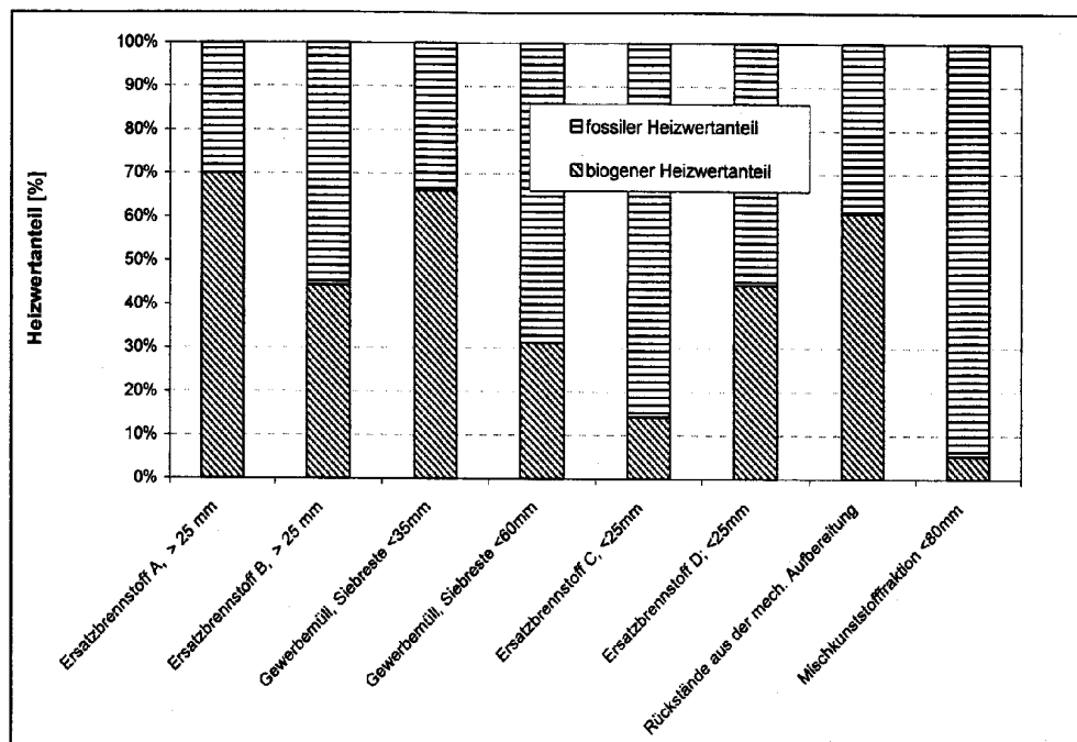
Fig. 3 biogener und fossiler Heizwertanteil [%] der Ersatzbrennstoffe
