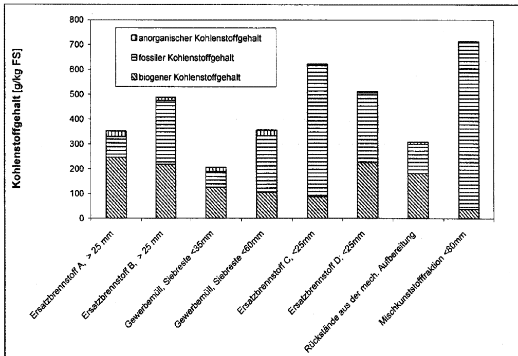
Fig. 2 Kohlenstoffgehalte [g/kg FS] der Ersatzbrennstoffe (unterteilt in biogenen, fossilen und anorganischen Kohlenstoff)
