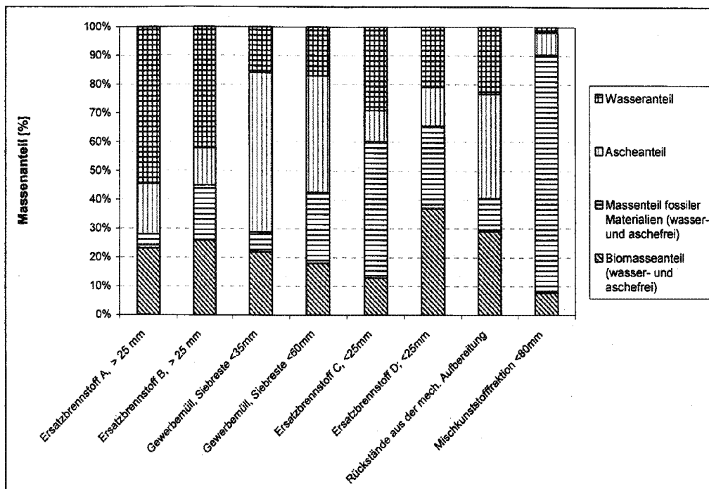
Fig. 1 Massenanteile biogener, fossiler und inerter Materialien, sowie der Wassergehalt der Ersatzbrennstoffe (Biogene und fossile Materialien beinhalten nur die wasser- und aschefreie organische Substanz)
