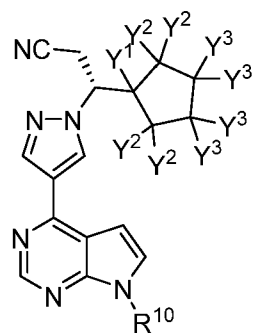
(IV)
