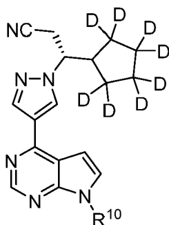
(IV A)
