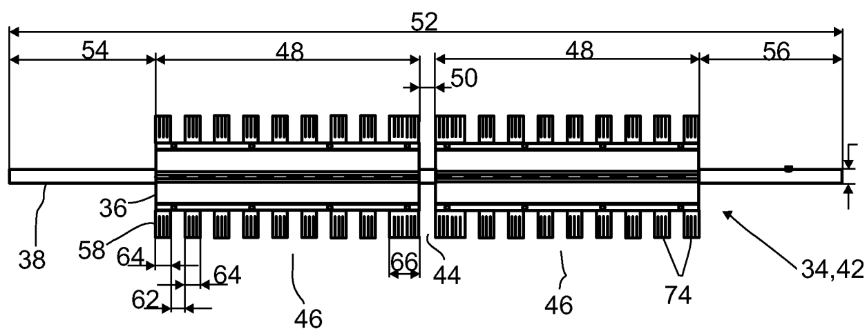
FIG.3 A-A
