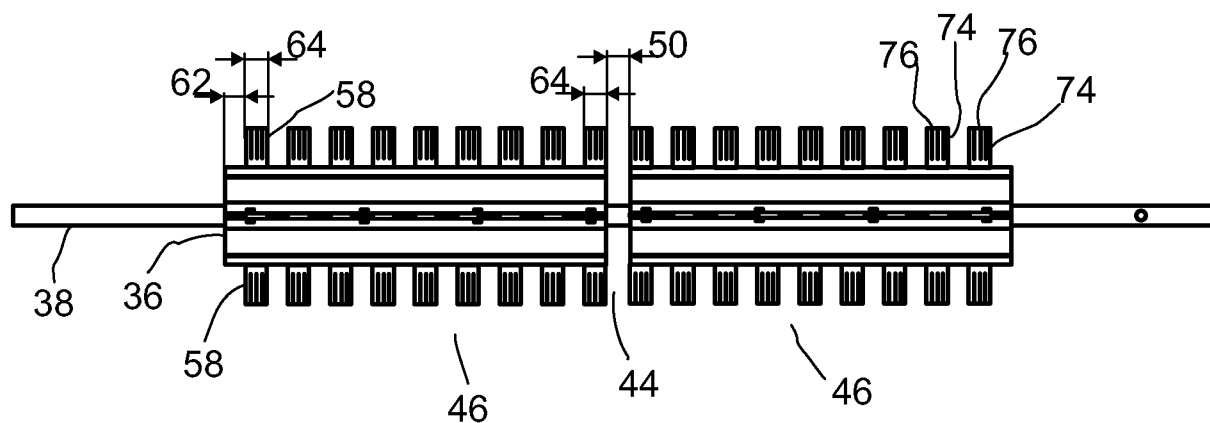
FIG.4 B-B
