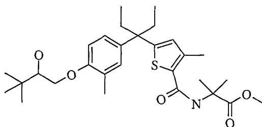
Enantiomer 1
