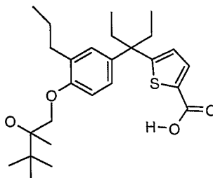
enantiomer 1
