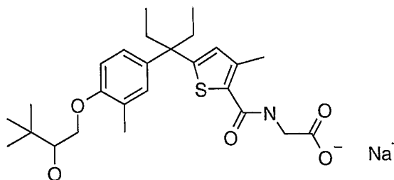
Enantiomer 1
