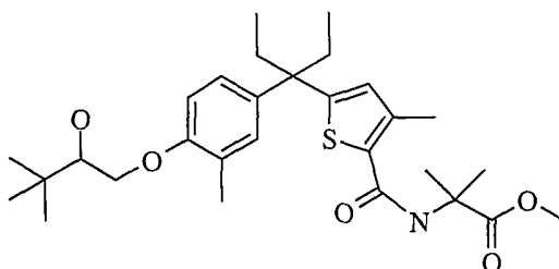
Enantiomer 2
