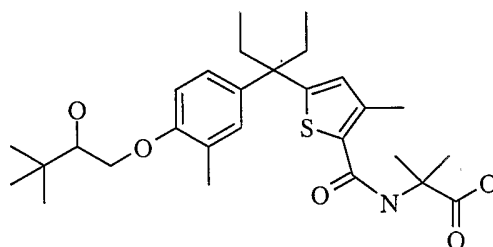
Enantiomer 1
