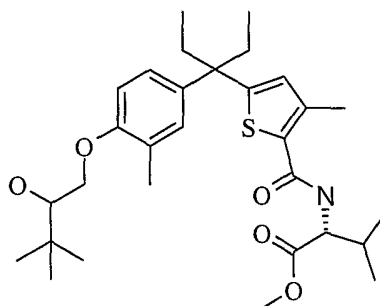
D -Racemic
