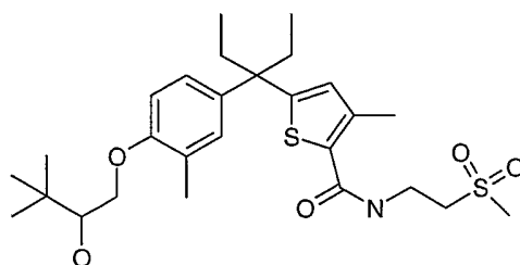
Enantiomer 1
