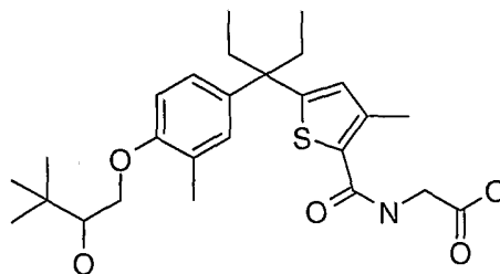
Enantiomer 2
