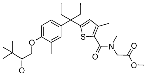
Enantiomer-2
