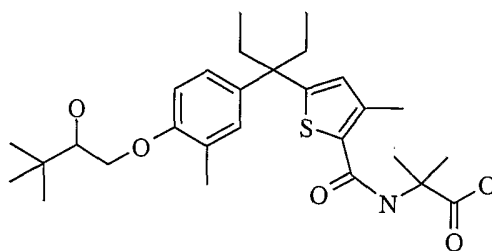
Enantiomer 2
