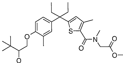
Enantiomer 1
