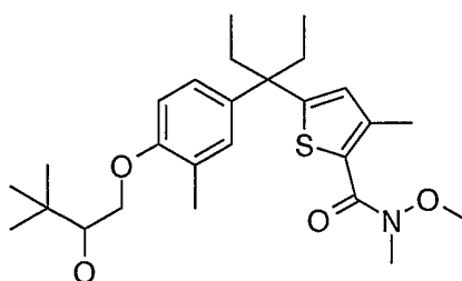
Enantiomer 2
