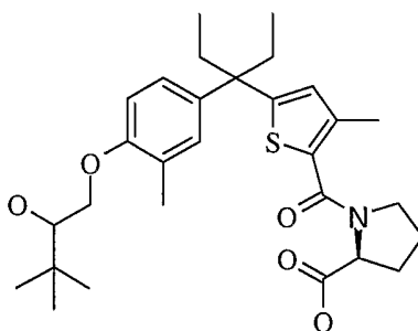
L -Enantiomer 1
