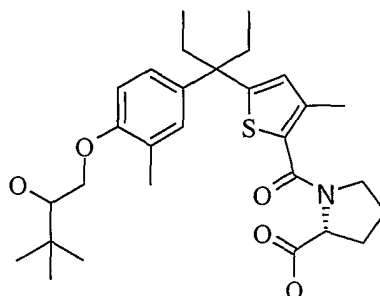
D -Enantiomer 2
