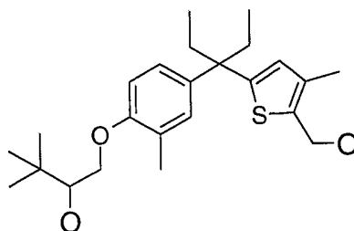
Enantiomer 2
