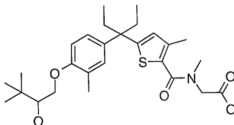
Enantiomer 2
