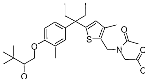
Enantiomer 1
