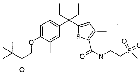
Enantiomer 2
