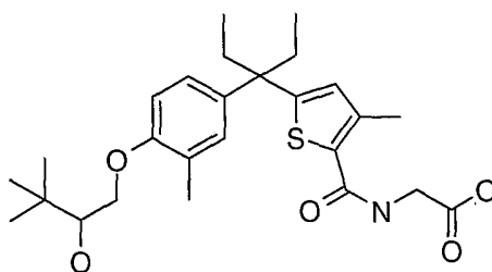
Enantiomer 1
