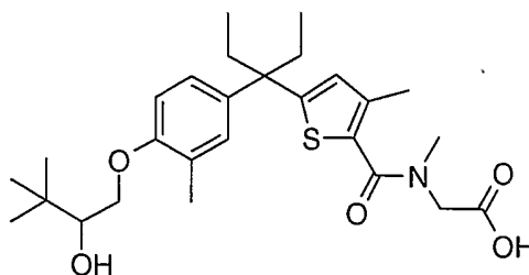
Enantiomer 1
