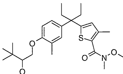
Enantiomer1
