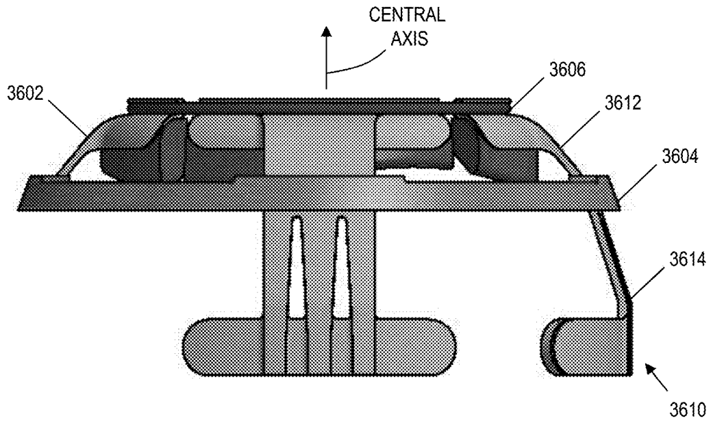
(SIDE) 3600 FIG. 36A
