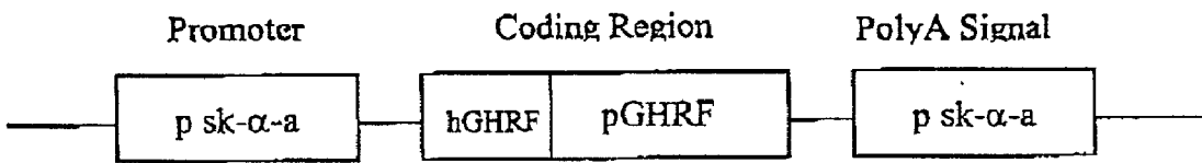
A. pUPAGRF
