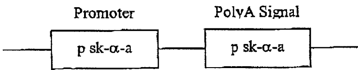
B. pUPAX
