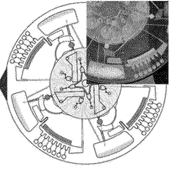
단계 #4. 세척용액을 폐기물 챔버로 옮긴다
