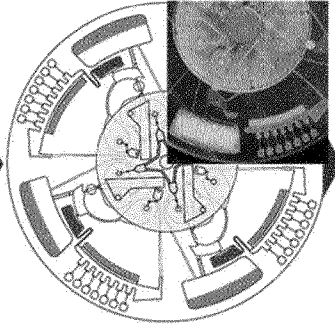
단계 #11. 왁스를 녹여 반응챔버를 밀봉한다
