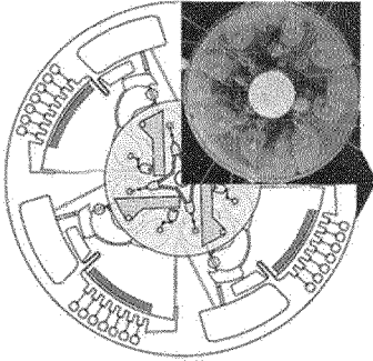
단계 #6. 정제된 RNA와 RT-LAMP 마스터 믹스를 수집챔버로 옮긴다
