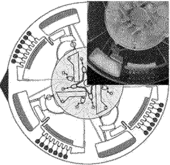
단계 #10. 7개의 반응챔버에 혼합물을 분취한다
