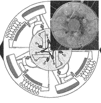
단계 #5. 용리용액과 RT-LAMP 마스터 믹스를 주입한다
