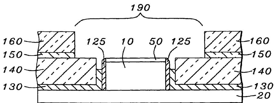
FIG. 6h
