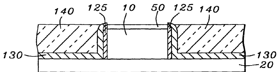
FIG. 6g
