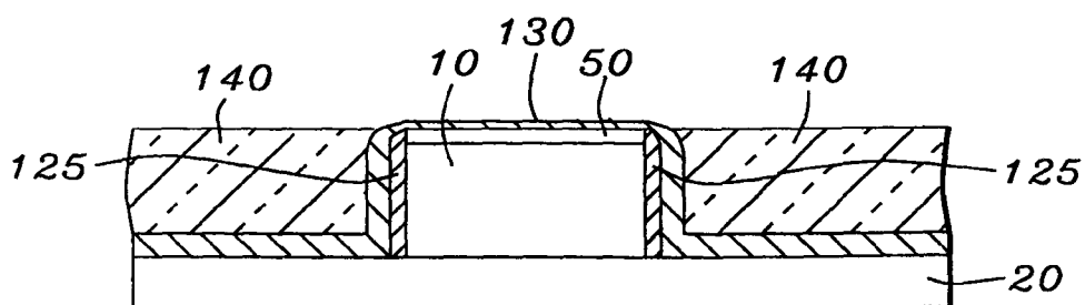
FIG. 6f
