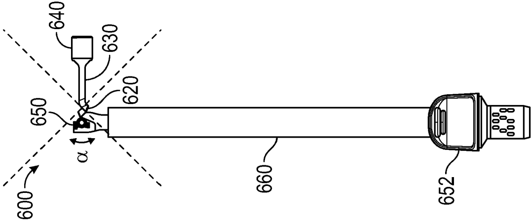
FIG. 6D
