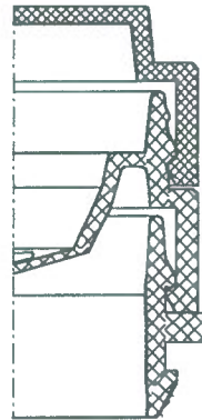
Szczegół 'A'
