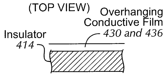
FIG. 4E
