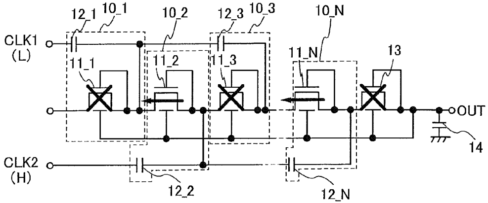
FIG. 5C T_CLKOFF
