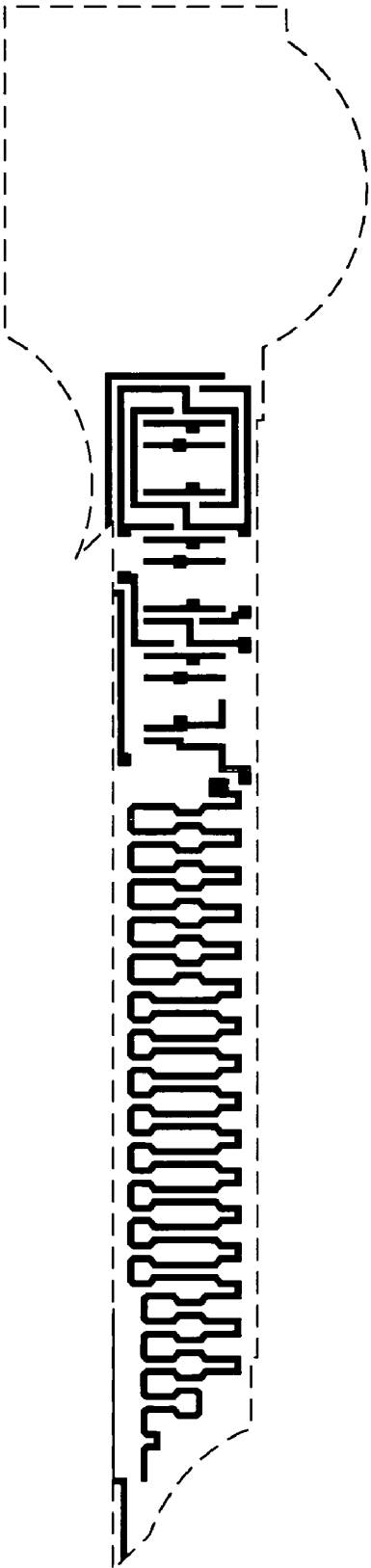
Poly mask
