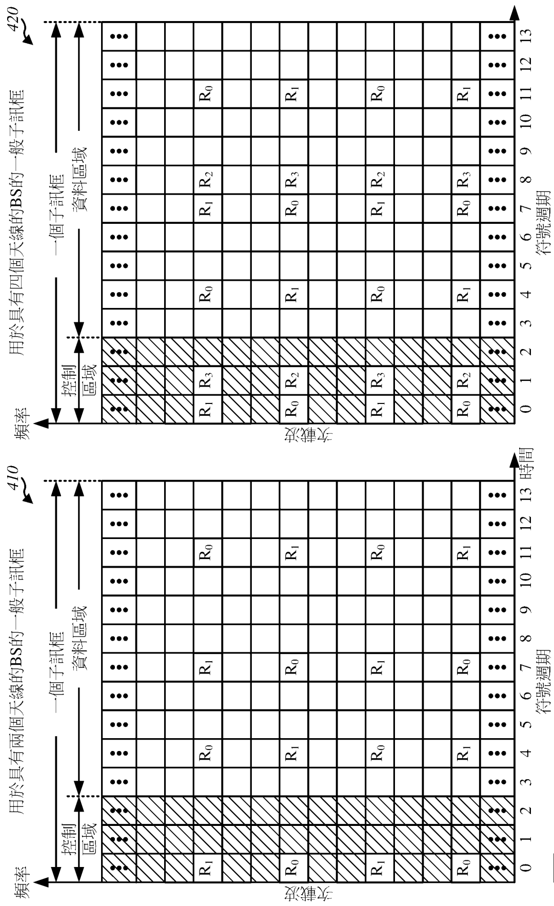
圖4 用於天線a的參考符號
