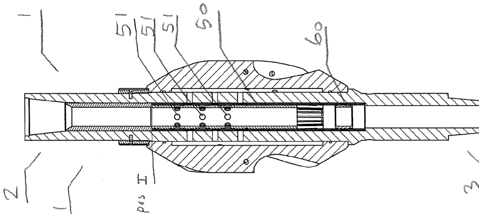
D-D(1:8)
