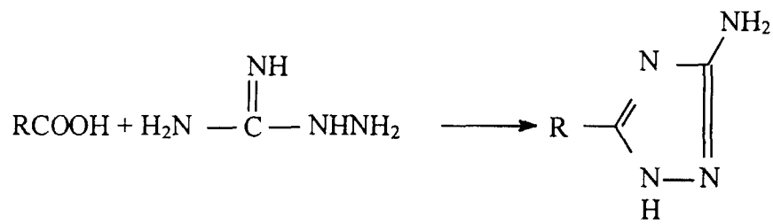
3-aminotriazole
