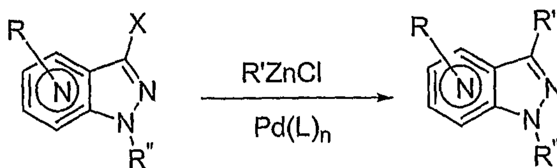
Scheme 1G
