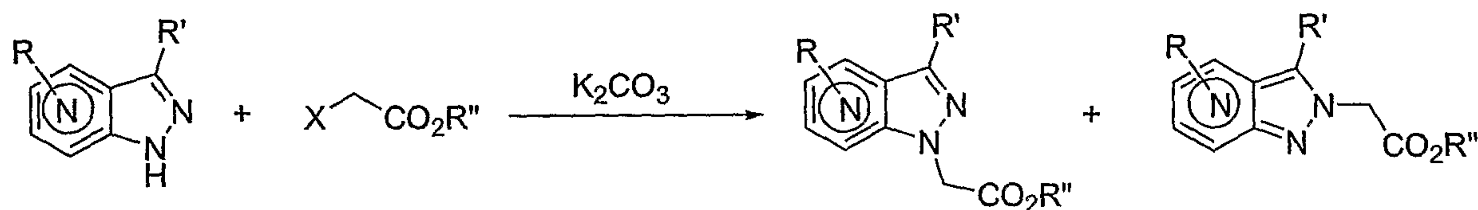
Scheme 1E
