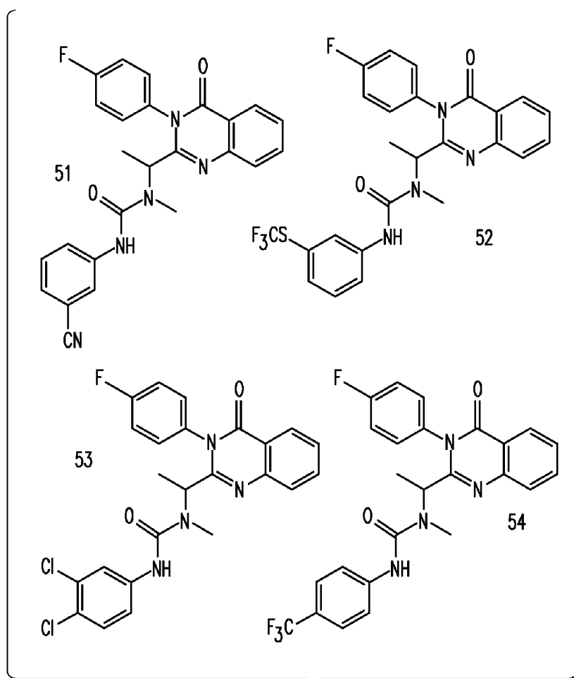
FIG.32F
