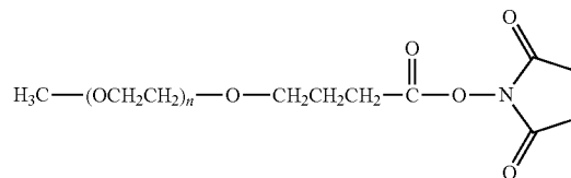
mPEG-Succinimidyl Butanoate
