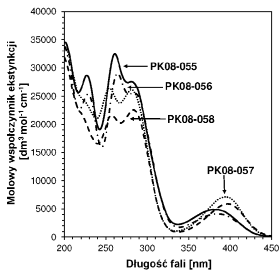
Wykres 2. Przykładowe widma absorpcji pochodnych 2-amino-4,6-difenylo-benzono-1,3-dikarbonitrylu.
