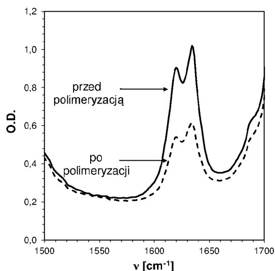
Wykres 3 Zmiana widma FT-IR dla monomeru akrylanowego TMPTA przed i po procesie fotopolimeryzacji rodnikowej przy naświetlaniu diodą UV-LED 405 nm w obecności związku PK02-071 (0,5%).
