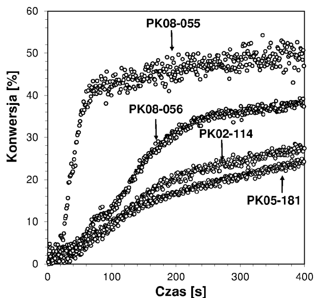
Wykres 6 Przykładowe profile kinetyczne przedstawiające przebieg fotopolimeryzacji monomerów BisGMA/TEGDMA(7:3) w obecności inicjatorów terfenylowych podczas naświetlania diodą LED 405 nm.
