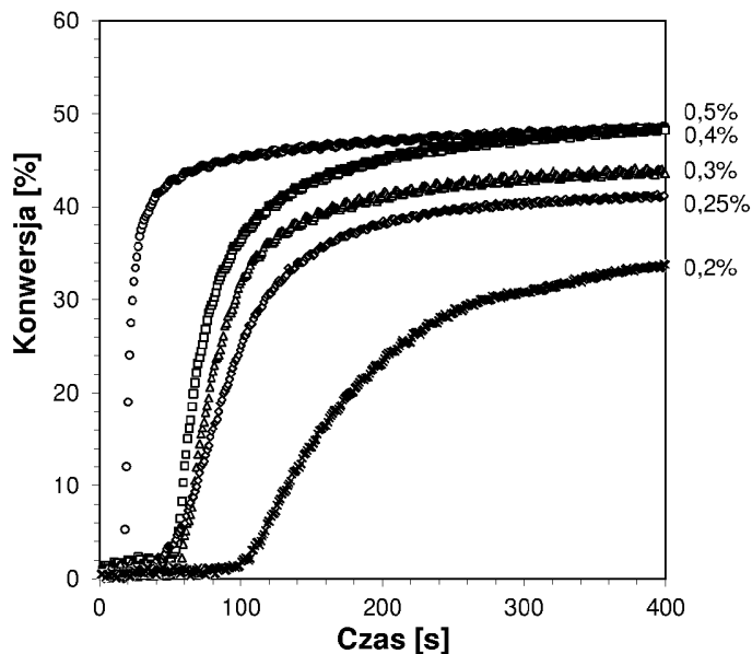
Wykres 5 Profile kinetyczne przedstawiające przebieg fotopolimeryzacji rodnikowej monomeru akrylanowego TMPTA w obecności różnych zawartości inicjatora PK08-060 podczas naświetlania diodą LED 405 nm.
