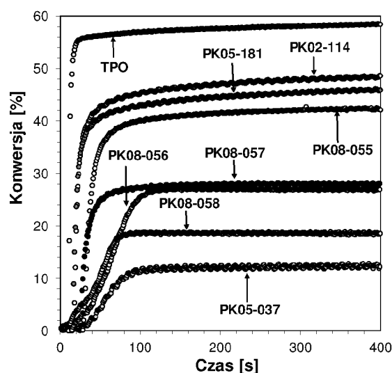
Wykres 4 Wybrane profile kinetyczne przedstawiające przebieg fotopolimeryzacji rodnikowej monomeru akrylanowego TMPTA w obecności inicjatorów terfenylowych podczas naświetlania diodą LED 405 nm.
