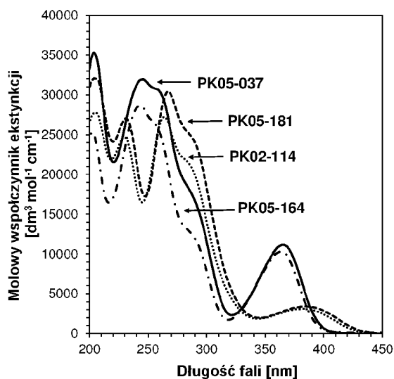
Wykres 1. Przykładowe widma absorpcji pochodnych 2-amino-4,6-difenylo-benzono-1,3-dikarbonitrylu.
