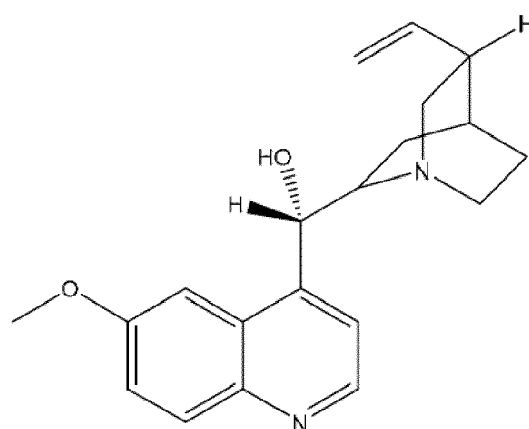
(VII)
