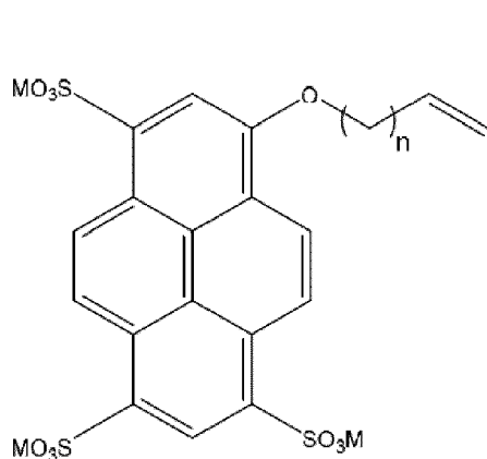
(VIII)
