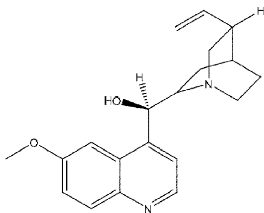
(VI)
