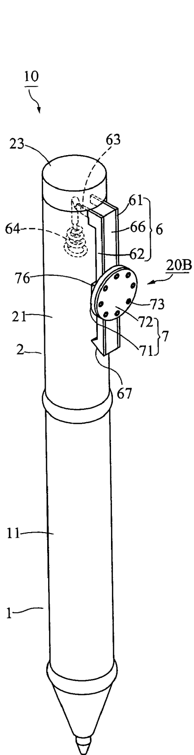
FIG. 8
