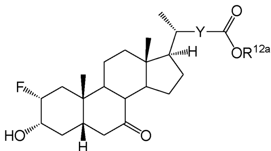
(XIIb)
