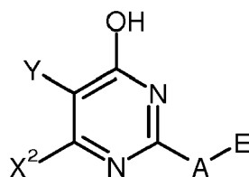
(XIb) ,
