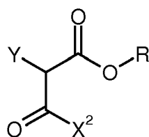
(IXb) ,
