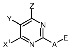
(IIId) ,
