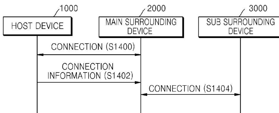
FIG. 14A
