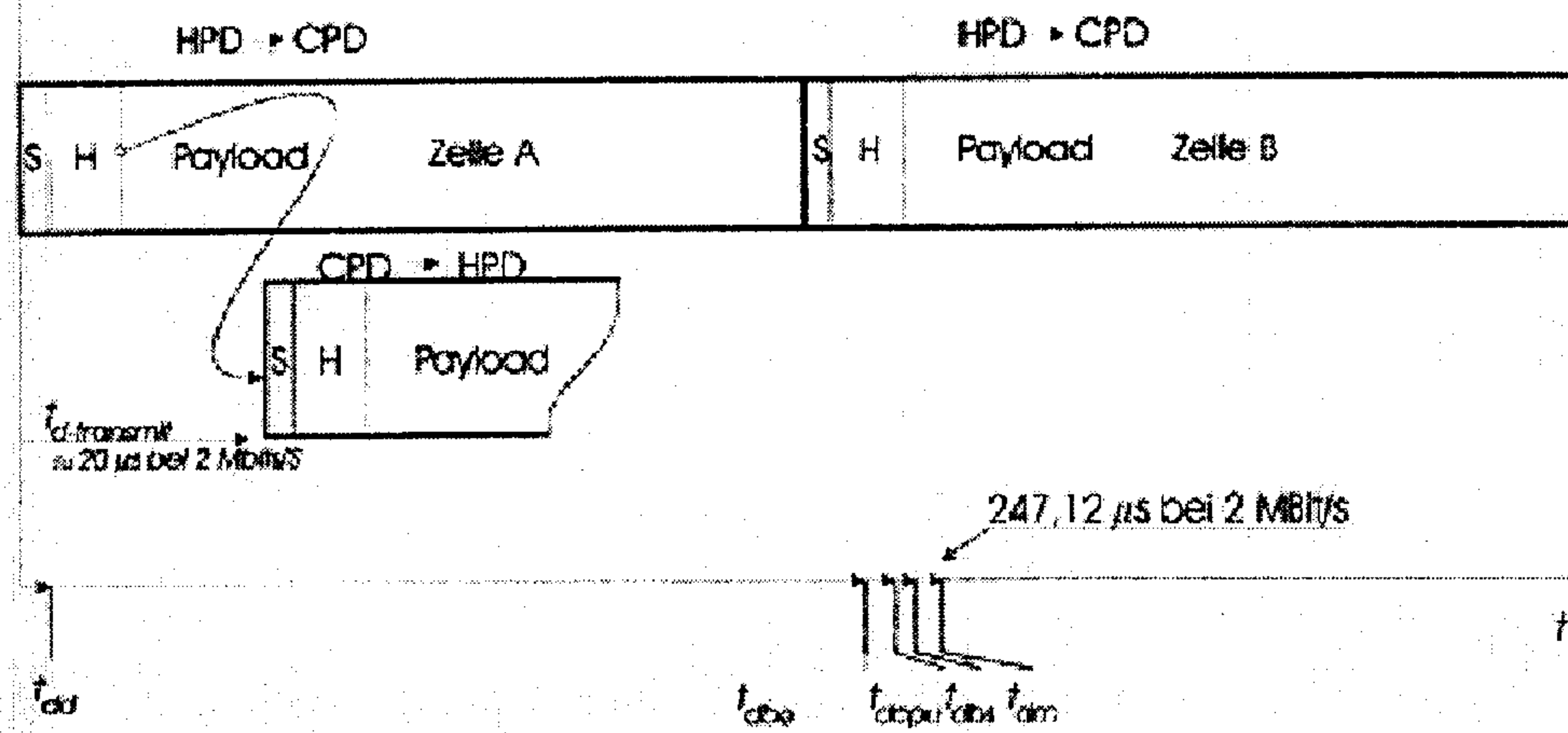
Abbildung 11: Sendesynchronisation und Verzögerungszeiten
