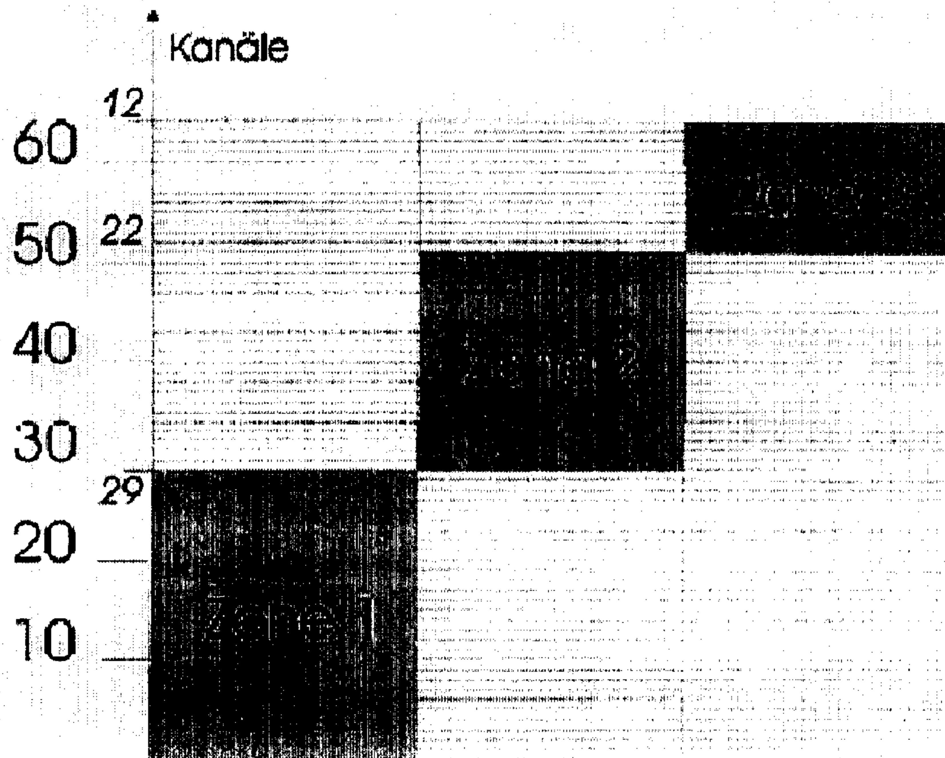
Abbildung 9: Bandbreitebereitstellung in den verschiedenen Zonen in Abhängigkeit von den aktiven SU-Kanälen
