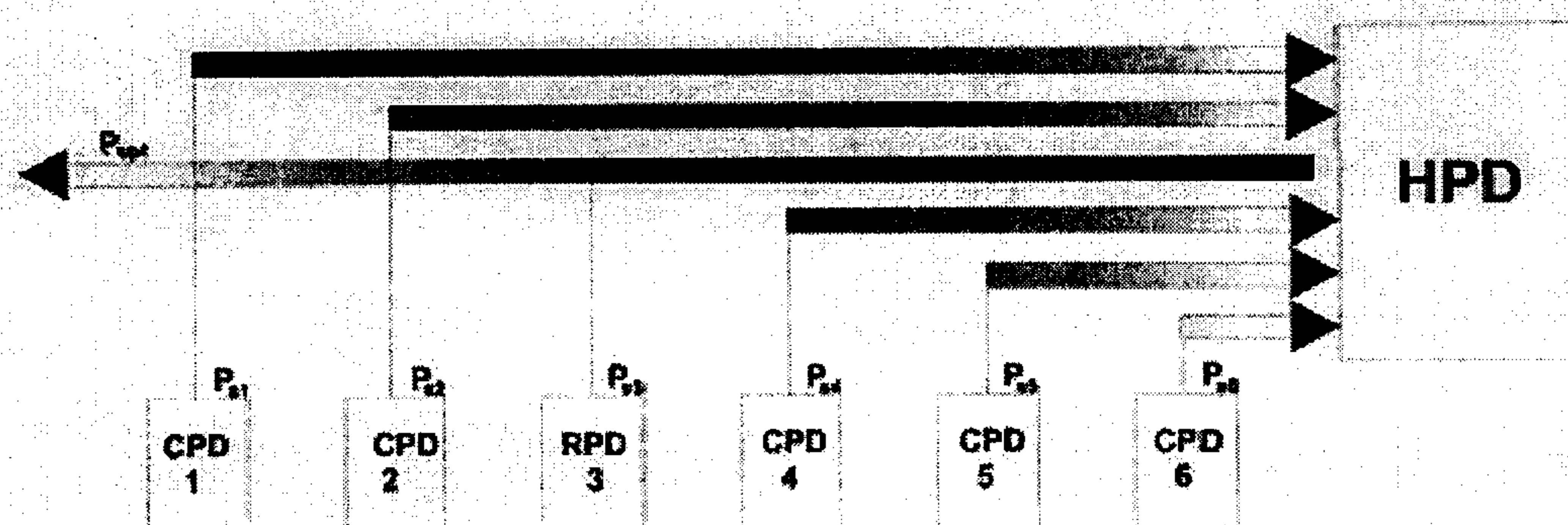
Abbildung 14: Optimale Sendeleistung und Repeaterauswahl
