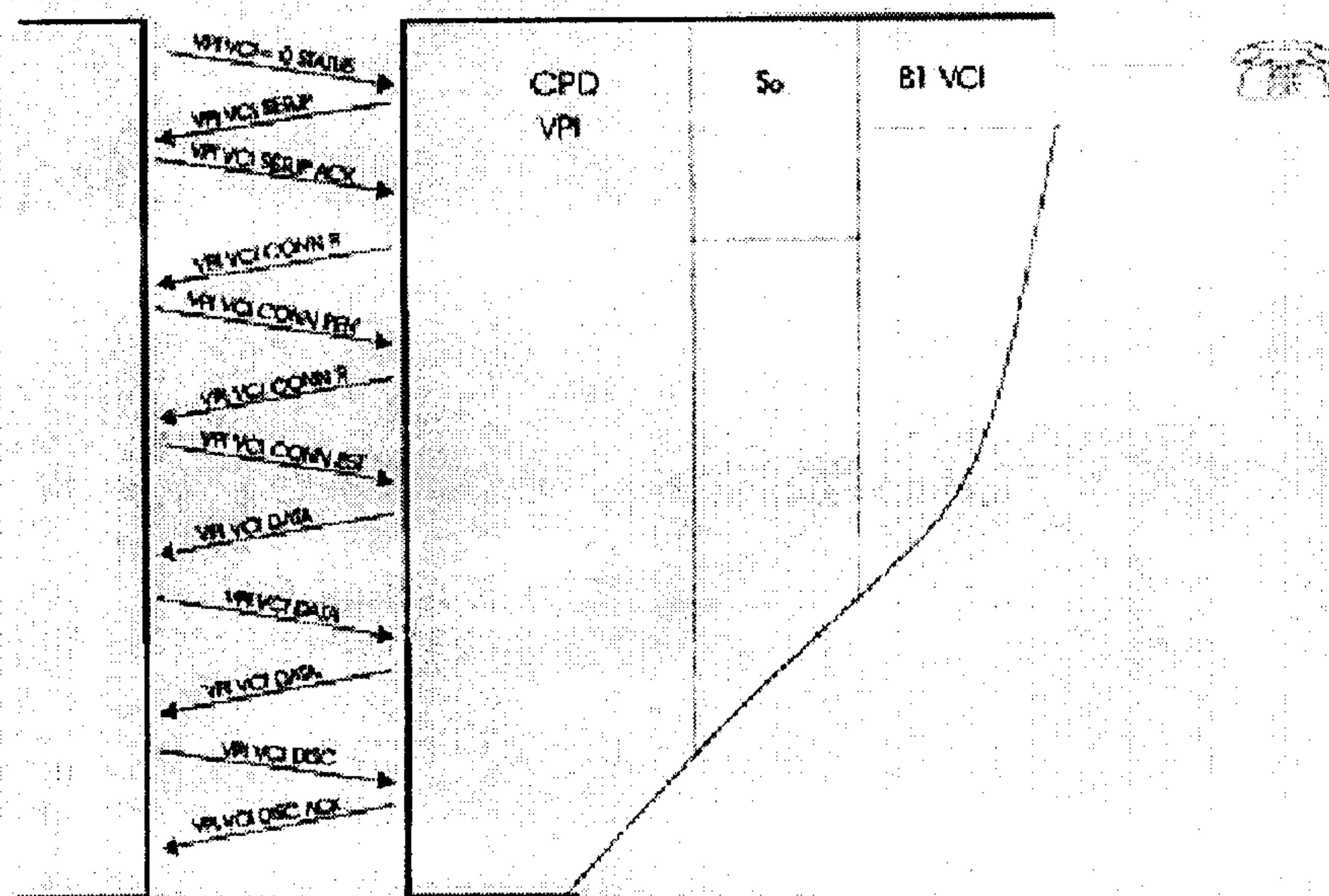
Abbildung 7: Verbindungsablauf, eine SU fordert die Verbindung an.
