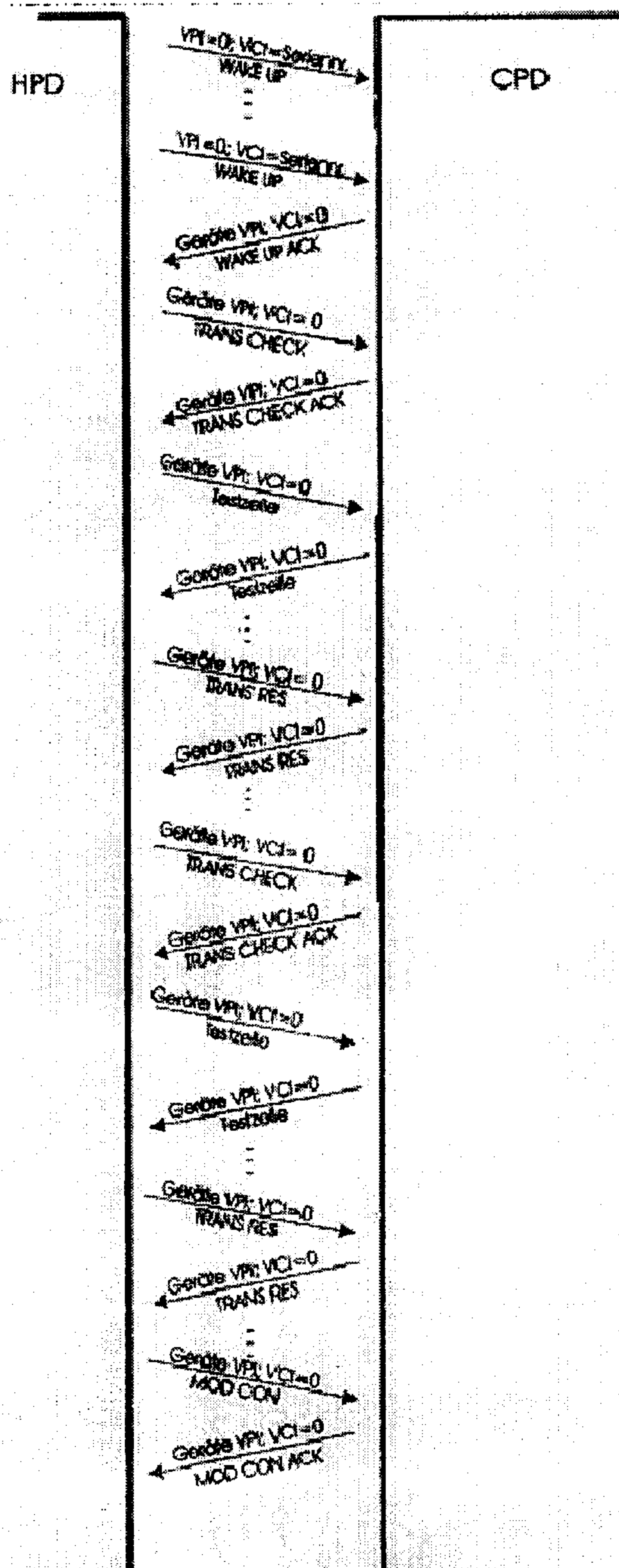
Abbildung 13: Signalisierung zur Inbetriebnahme eines CPD
