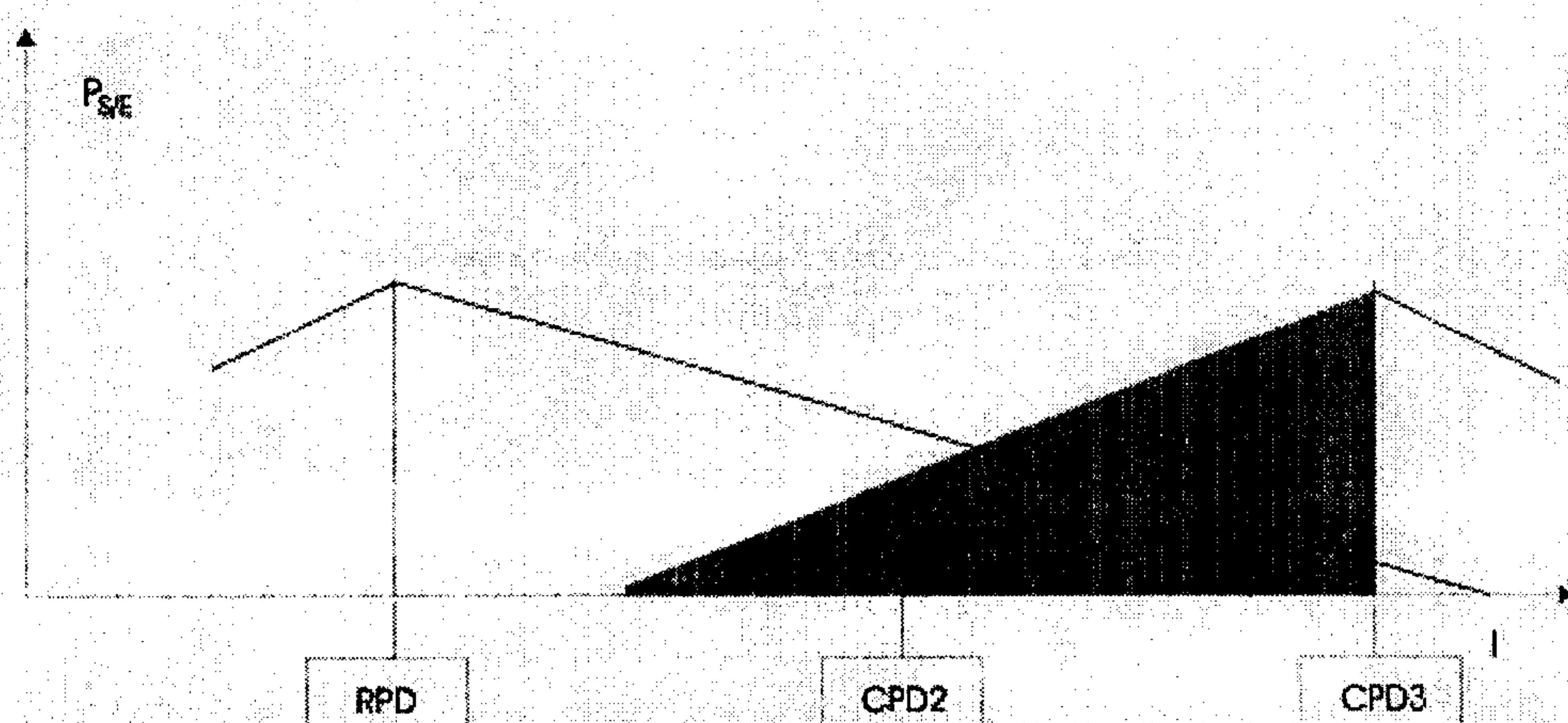
Abbildung 8: Problem der Mehrfachausnutzung von Leitungslagen
