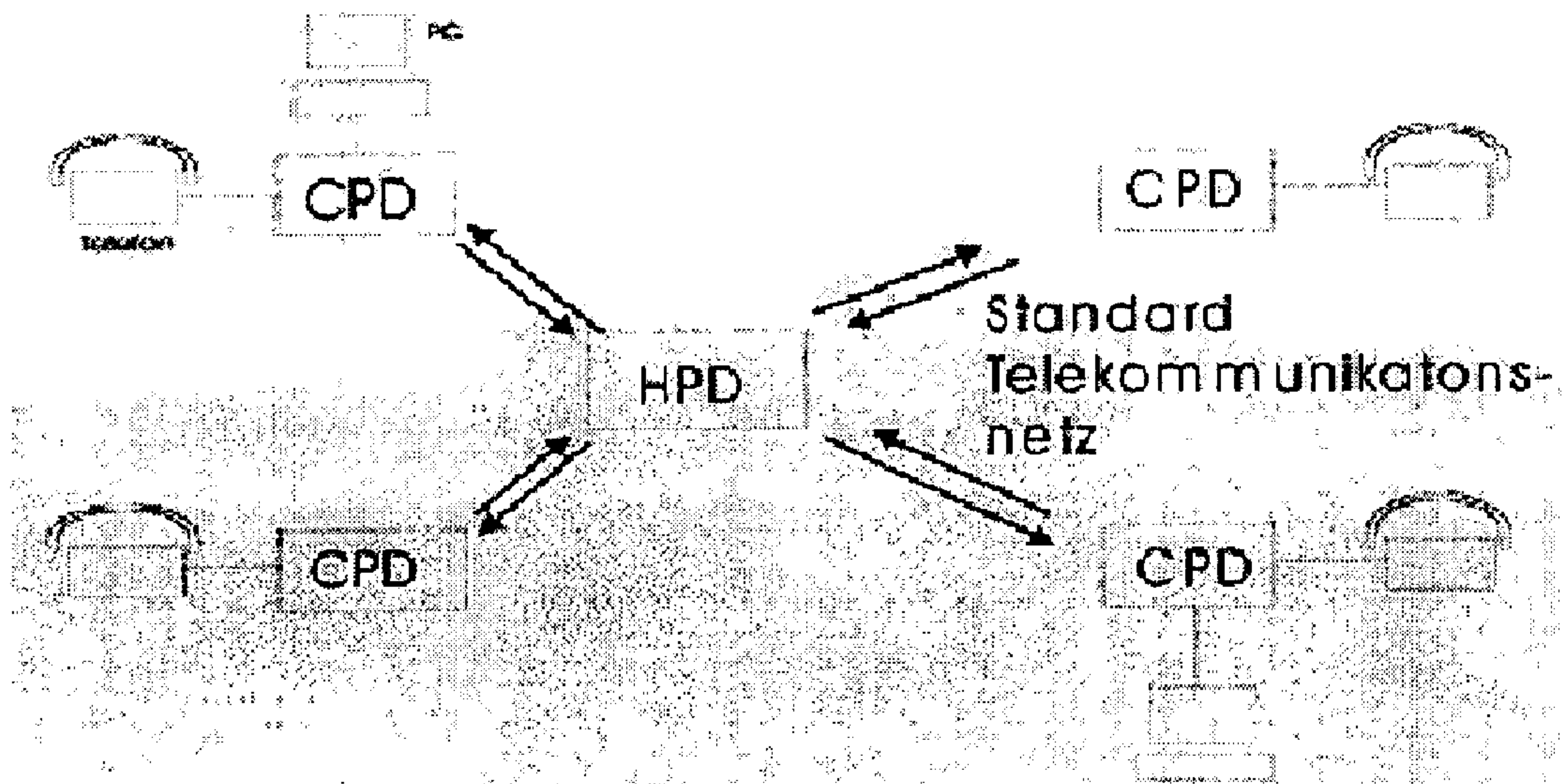
Abbildung 1: Das powerline Netz als logischer Stern
