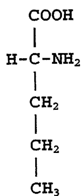
norvaline
