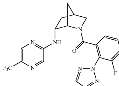
(3-fluoro-2-(2H-1,2,3-triazol-2-yl)phenyl)((1S,4S,6R)-6-((5-(trifluoromethyl)pyrazin-2-yl)amino)-2-azabicyclo[2.2.1]heptan-2-yl)methanone
