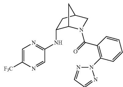
(2-((2H-1,2,3-triazol-2-yl)phenyl)((1S,4S,6R)-6-((5-(trifluoromethyl)pyrazin-2-yl)amino)-2-azabicyclo[2.2.1]heptan-2-yl)methanone
