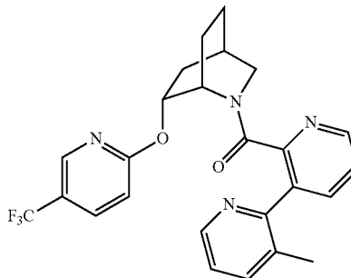
Example 599
