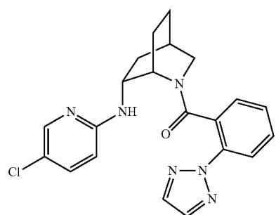
(2-(2H-1,2,3-triazol-2-yl)phenyl)((1S,4R,6R)-6-((5-chloropyridin-2-yl)amino)-2-azabicyclo[2.2.2]octan-2-yl)methanone
