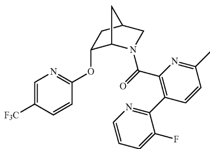
Example 344
