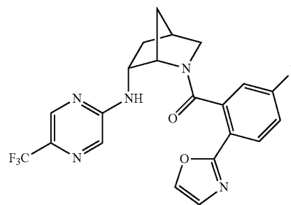
(5-fluoro-2-(oxazol-2-yl)phenyl)((1S,4S,6R)-6-((5-(trifluoromethyl)pyrazin-2-yl)amino)-2-azabicyclo[2.2.1]heptan-2-yl)methanone
