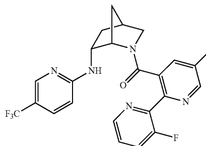
Example 396
