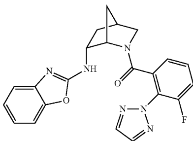
((1S,4S,6R)-6-(benzo[d]oxazol-2-ylamino)-2-azabicyclo[2.2.1]heptan-2-yl)(3-fluoro-2-(2H-1,2,3-triazol-2-yl)phenyl)methanone
