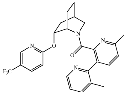
Example 596
