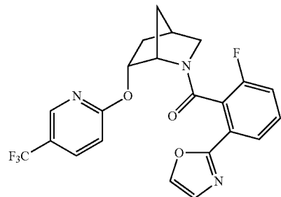
(2-fluoro-6-(oxazol-2-yl)phenyl)((1S,4R,6R)-6-((5-(trifluoromethyl)pyridin-2-yl)oxy)-2-azabicyclo[2.2.1]heptan-2-yl)methanone
