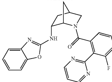
((1S,4S,6R)-6-(benzo[d]oxazol-2-ylamino)-2-azabicyclo[2.2.1]heptan-2-yl)(3-fluoro-2-(pyrimidin-2-yl)phenyl)methanone
