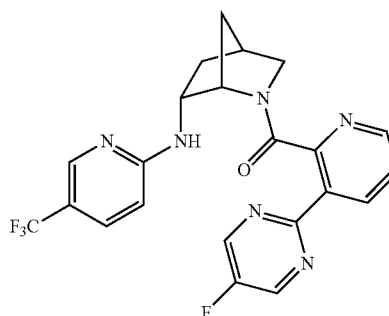
Example 377
