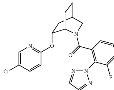
Example 479
