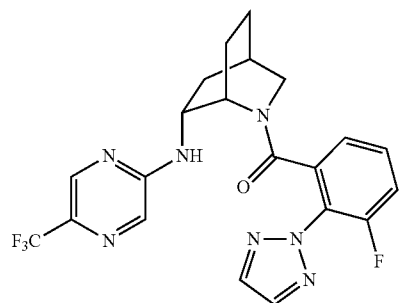
(3-fluoro-2-(2H-1,2,3-triazol-2-yl)phenyl)((1S,4R,6R)-6-((5-(trifluoromethyl)pyrazin-2-yl)amino)-2-azabicyclo[2.2.2]octan-2-yl)methanone
