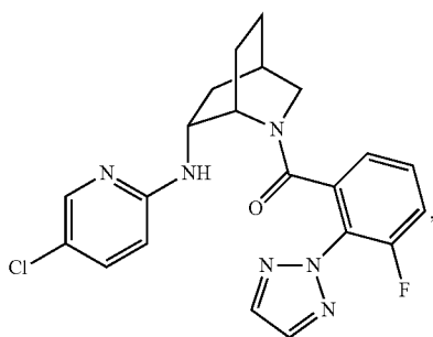
((1S,4R,6R)-6-((5-chloropyridin-2-yl)amino)-2-azabicyclo[2.2.2]octan-2-yl)(3-fluoro-2-(2H-1,2,3-triazol-2-yl)phenyl)methanone
