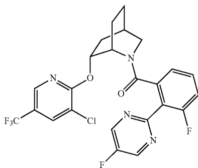
Example 445
