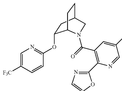
Example 611
