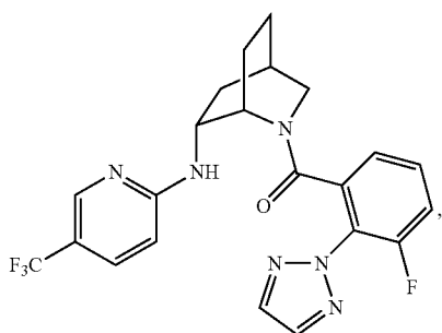
(3-fluoro-2-(2H-1,2,3-triazol-2-yl)phenyl)((1S,4R,6R)-6-((5-(trifluoromethyl)pyridin-2-yl)amino)-2-azabicyclo[2.2.2]octan-2-yl)methanone
