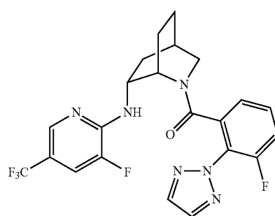
(3-fluoro-2-(2H-1,2,3-triazol-2-yl)phenyl)((1S,4R,6R)-6-((3-fluoro-5-(trifluoromethyl)pyridin-2-yl)amino)-2-azabicyclo[2.2.2]octan-2-yl)methanone
