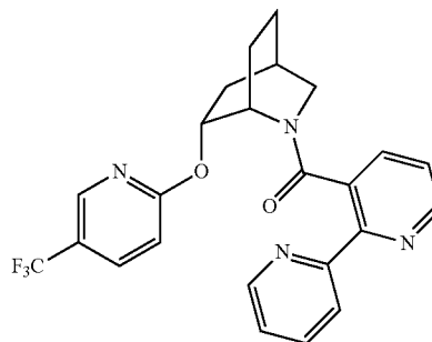
Example 593
