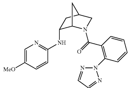
(2-(2H-1,2,3-triazol-2-yl)phenyl)((1S,4S,6R)-6-((5-(methoxypyridin-2-yl)amino)-2-azabicyclo[2.2.1]heptan-2-yl)methanone
