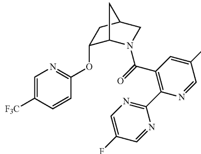
Example 324
