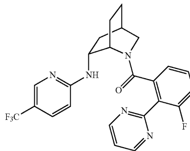
Example 502
