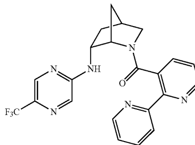
Example 635
