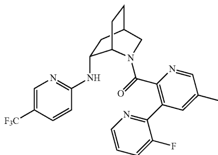
Example 393
