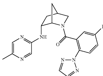
(5-fluoro-2-(2H-1,2,3-triazol-2-yl)phenyl)((1S,4S,6R)-6-((5-methylpyrazin-2-yl)amino)-2-azabicyclo[2.2.1]heptan-2-yl)methanone
