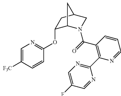
Example 327
