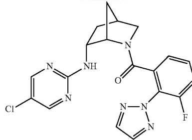
((1S,4S,6R)-6-((5-chloropyrimidin-2-yl)amino)-2-azabicyclo[2.2.1]heptan-2-yl)(3-fluoro-2-(2H-1,2,3-triazol-2-yl)phenyl)methanone
