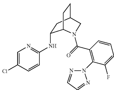
Example 523
