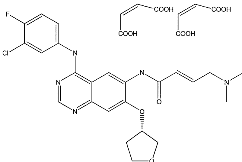
Afatinib
