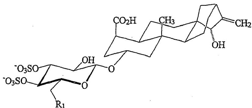
(IV)
