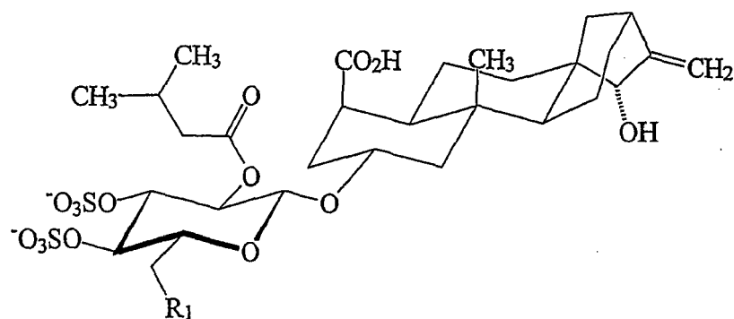
(II)
