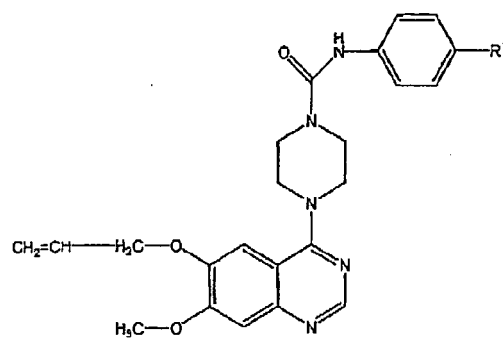
Formula I(d)
