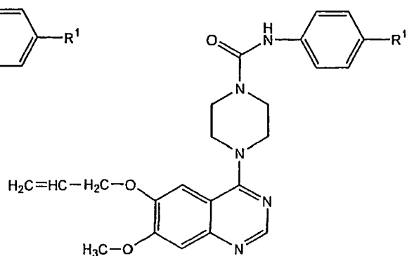
Formula I(d)
