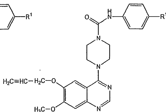
Formula I(d)
