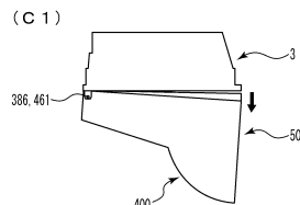
【図13-43】 開閉扉枠 [第1開状態 (開放角度: 約5度)]
