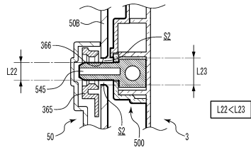
【図13-50】 球抜き通路 (特定内部進入部品と被進入部品)
