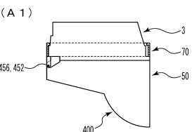
【図13-45】 遊技機用枠+開閉扉枠 [閉状態]
