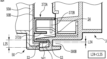
【図13-51】 開閉扉枠底部部品 (特定内部進入部品と被進入部品／ドア枠所定部品と内枠所定部品)
