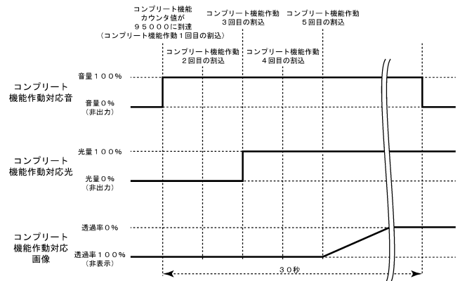
コンプリート機能作動時の出力タイミング
