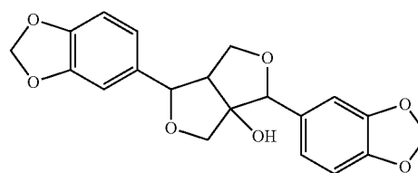
Paulownin
