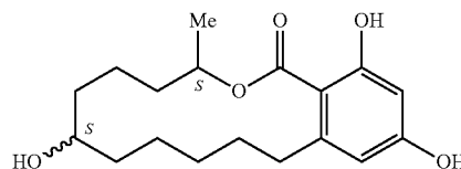
\beta -Zearalanol
