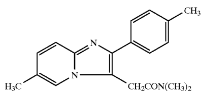
Zolpidem
