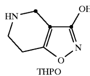
THPO
