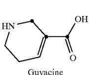
Guvacine
