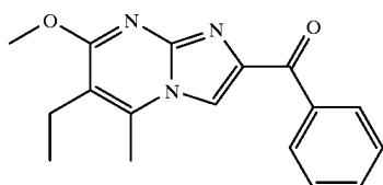
divaplon (RU32698)
