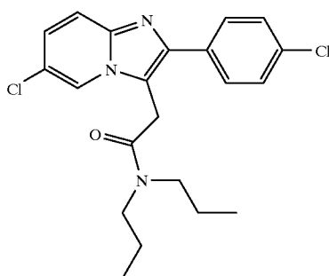
alpidem
