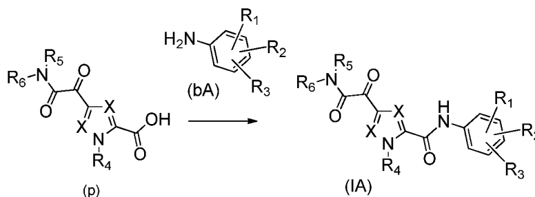
Scheme 2A
