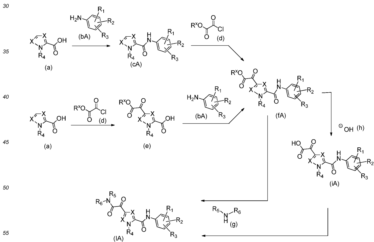
Scheme 1A
