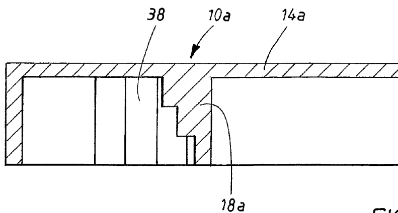
FIG. 4f A-A
