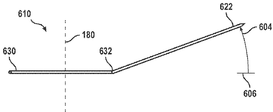
VIEW A-A FIG. 6B
