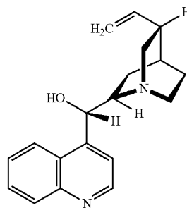
Cinchonine
