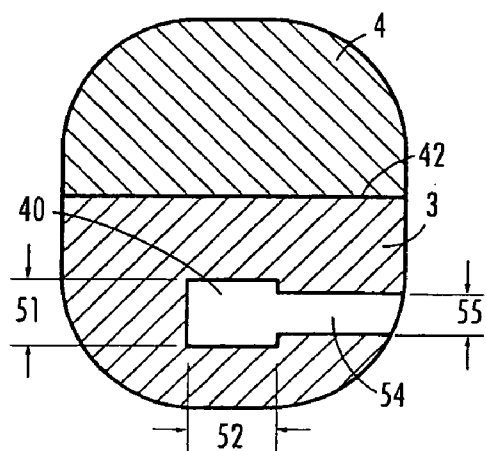
SEC A-A FIG. 5
